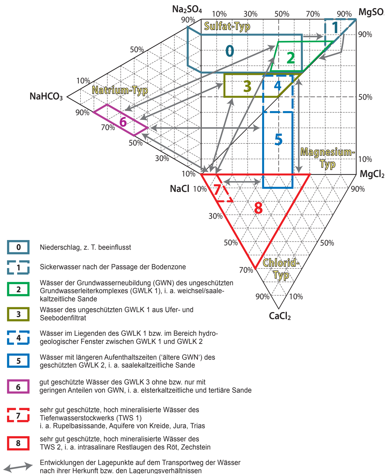
Abb.1 Hydrogeochemisches Genese-Modell der Wässer in den Grundwasserleiterkomplexen des Landes Brandenburg (RECHLIN 1997)
