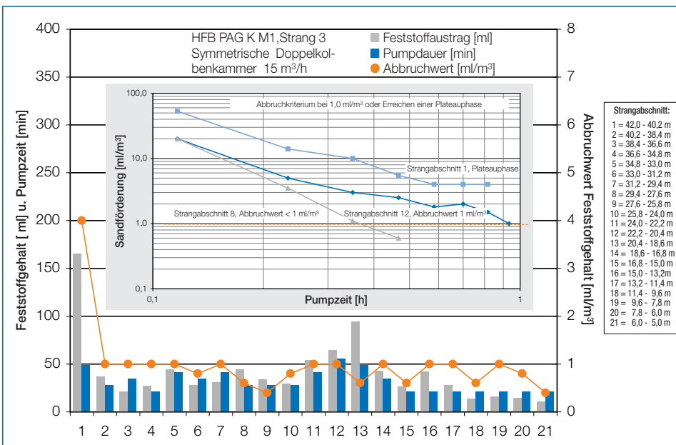
Abb. 3: Abschnittweise gemessene Werte für Pumpzeit, Feststoffaustrag und dessen Abbruchwert beim Test der symmetrischen Doppelkolbenkammer im Strang 3 des Horizontalfilterbrunnens Kapellen Mitte 1 im Anschluss an die Reinigung mittels Manschettenkammer und beispielhaft drei Feststoffaustragsmessungen
