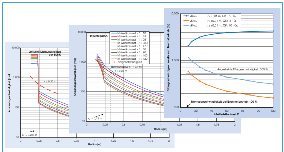
Abb. 4: Strömungsgeschwindigkeiten für verschiedene Durchlässigkeitskontrastwerte in Abhängigkeit von der radialen Entfernung von der Filterachse auf Höhe „Mitte Dichtungskolben“ und „Mitte offene Kammer“ der SDKK sowie erreichbare Filtergeschwindigkeiten in Prozent bezüglich Normalbetrieb 1 cm vor und 1 cm hinter der Bohrlochwand
